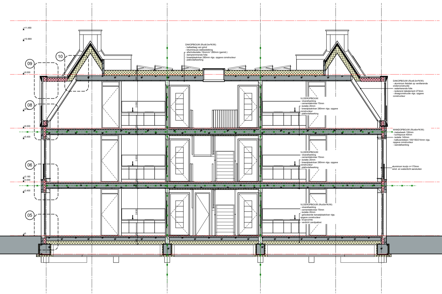
Doorsnede D-D
