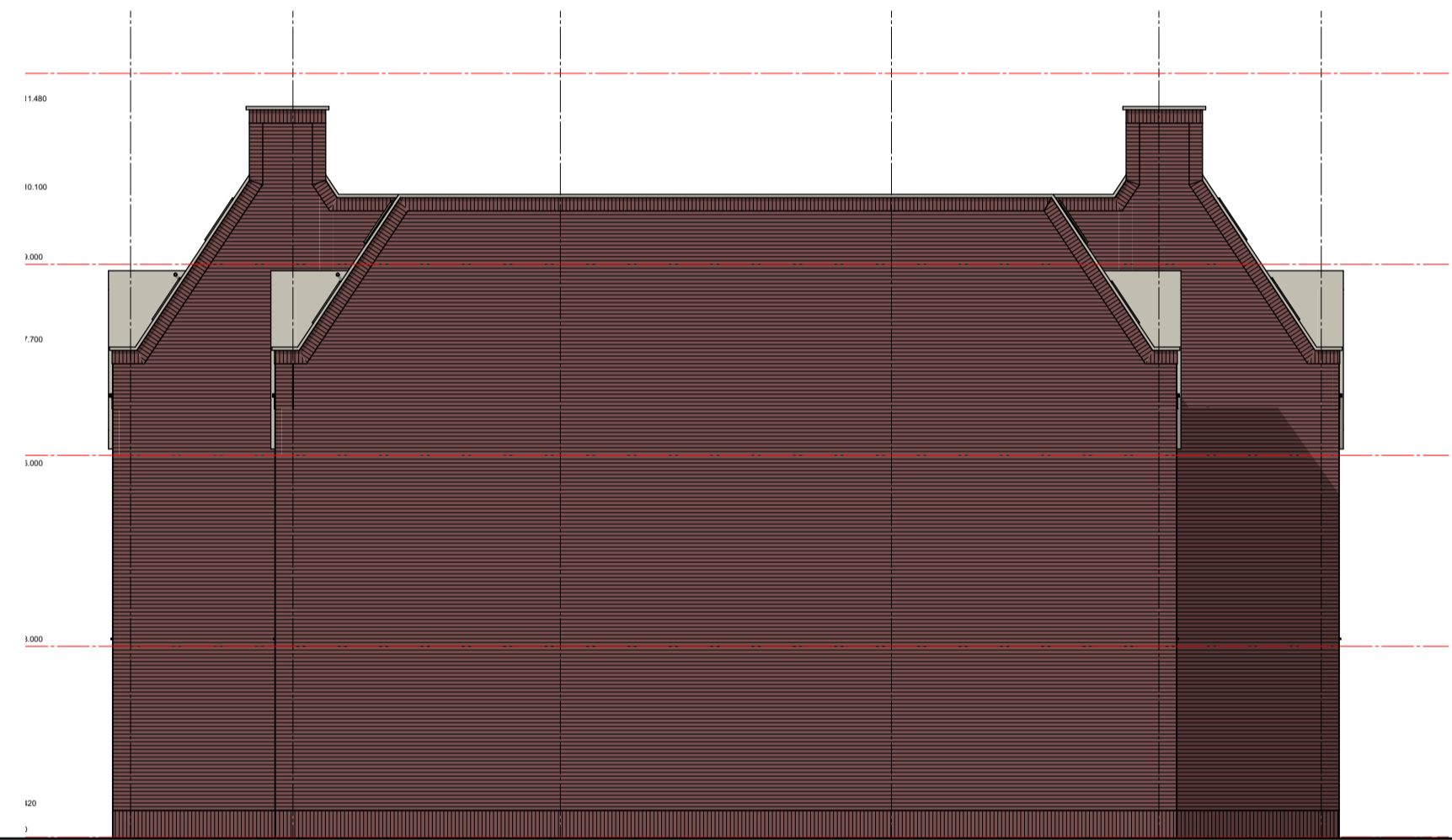
voorgevel
