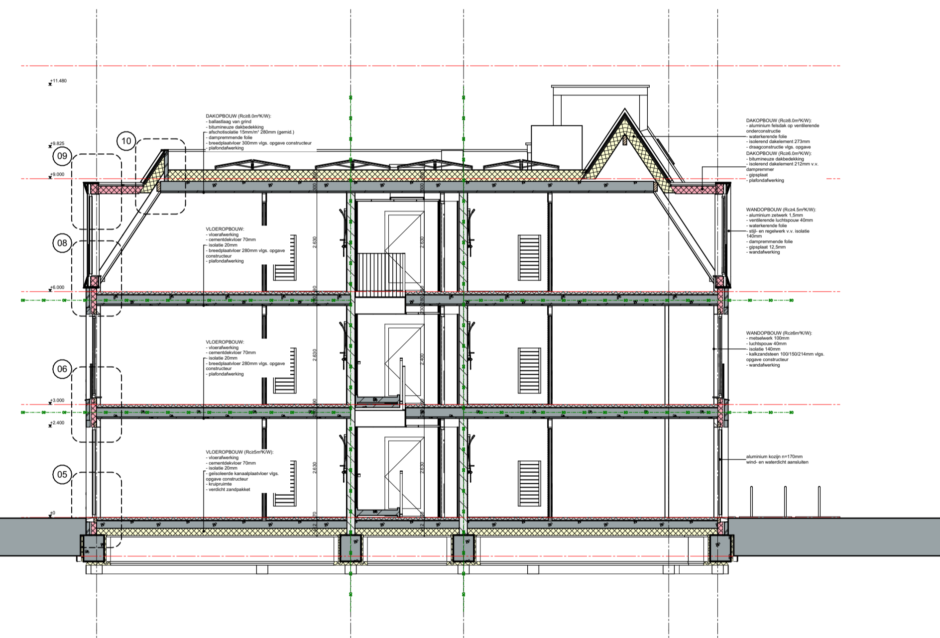
Doorsnede A-A
